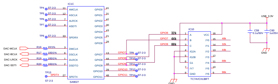
Audio_I/F
